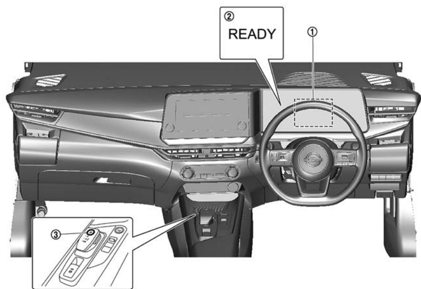
① アドバンスドドライブアシストディスプレイ ② 走行可能表示灯 ③ Pスイッチ
